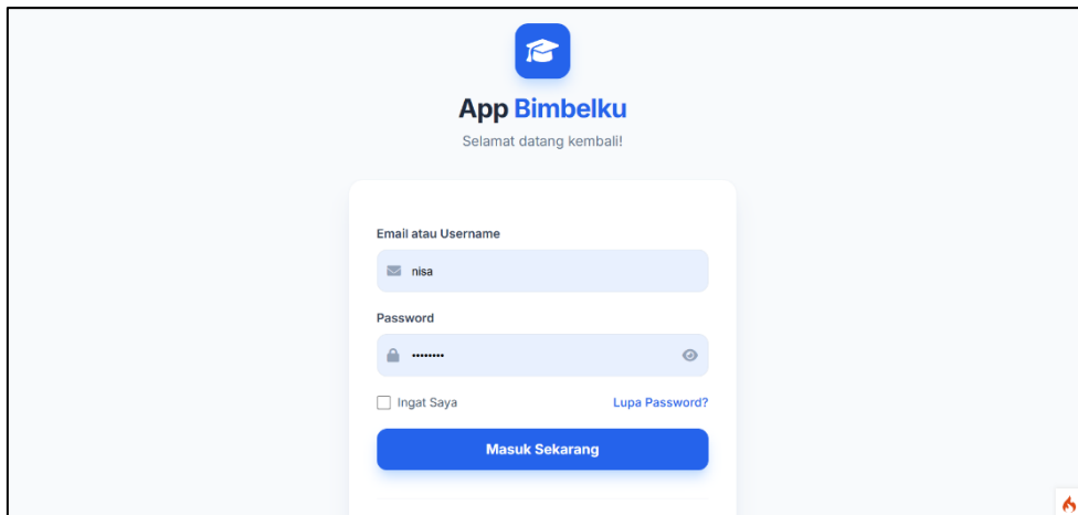
Gambar 4. Halaman Login
