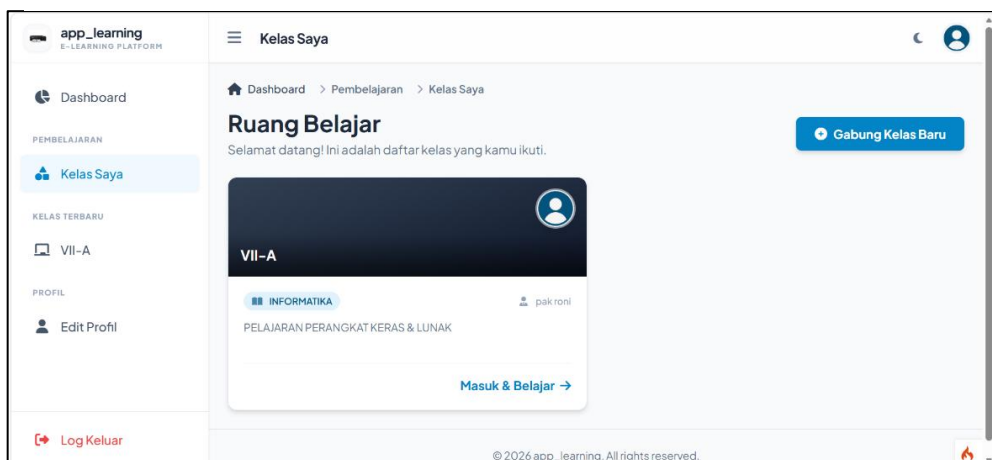
Gambar 5. Halaman Kelas
