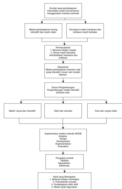
Gambar 3. Kerangka Berfikir
